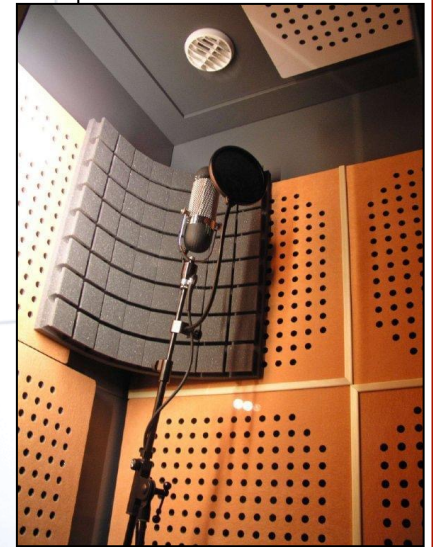
Studiobricks ONE, fungerar även som sångbås.
