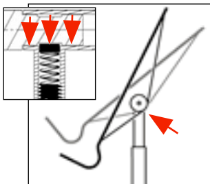
Exakt vinkelinställning av brättet med friktionslås med tryckbelastad stål fjäder.
