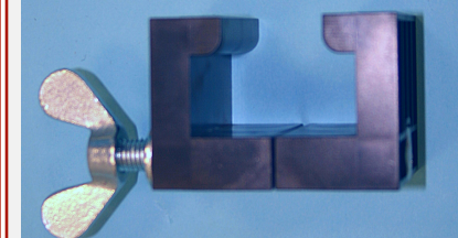
Podielås. Av plast eller stål. "Rådarnas favorit" p.g.a. den snabba kopplingen. Passar i spår på podieramens insida.
